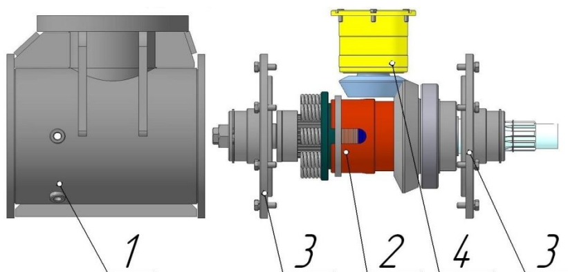
Рисунок 2. Общий вид и основные узлы Редуктора конического ФД-567.01
