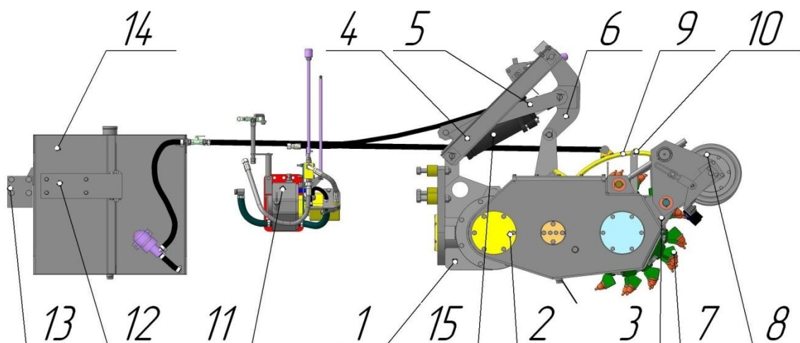
Рисунок 1. Общий вид и основные узлы Фрезы дорожной ФД-567
