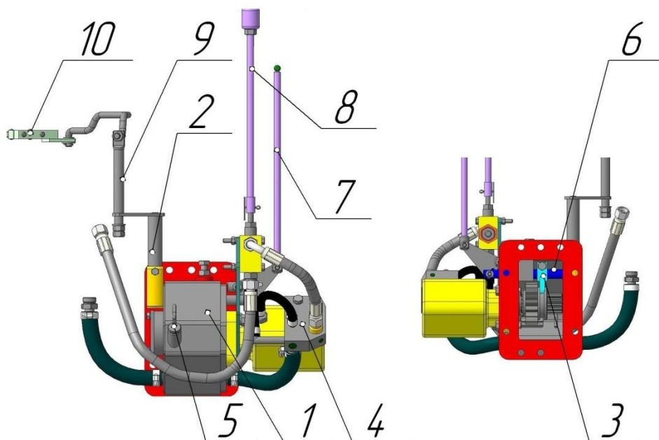
Рисунок 11. Общий вид и основные узлы Гидроходоуменьшителя ФД-567.11
