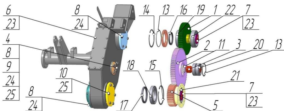
Рисунок 5. Редуктор цилиндрический ФД-567.02
