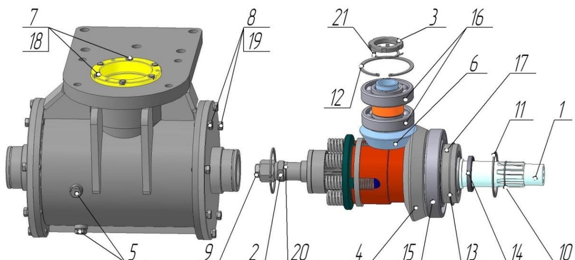
Рисунок 4. Редуктор конический ФД-567.01
