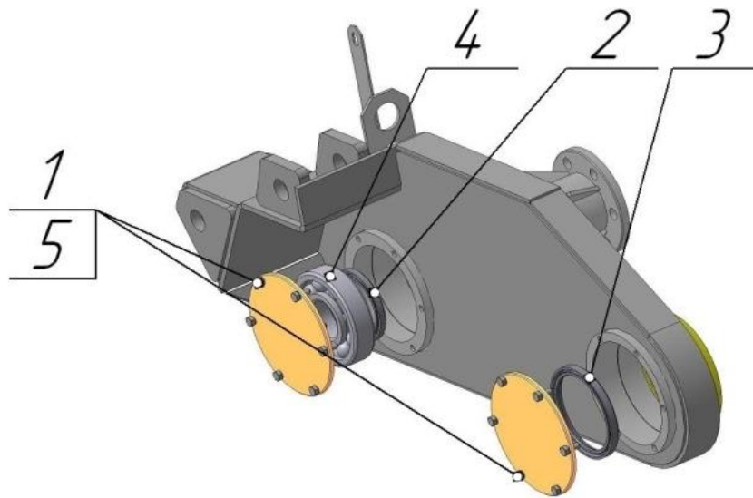
Рисунок 6. Опора ФД-567.03
