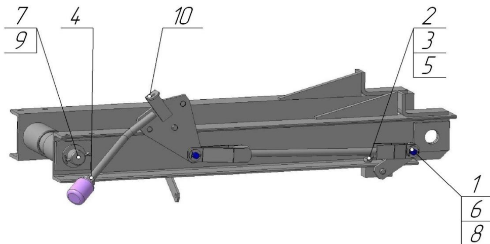
Рисунок 7. Рамка ФД-567.04
