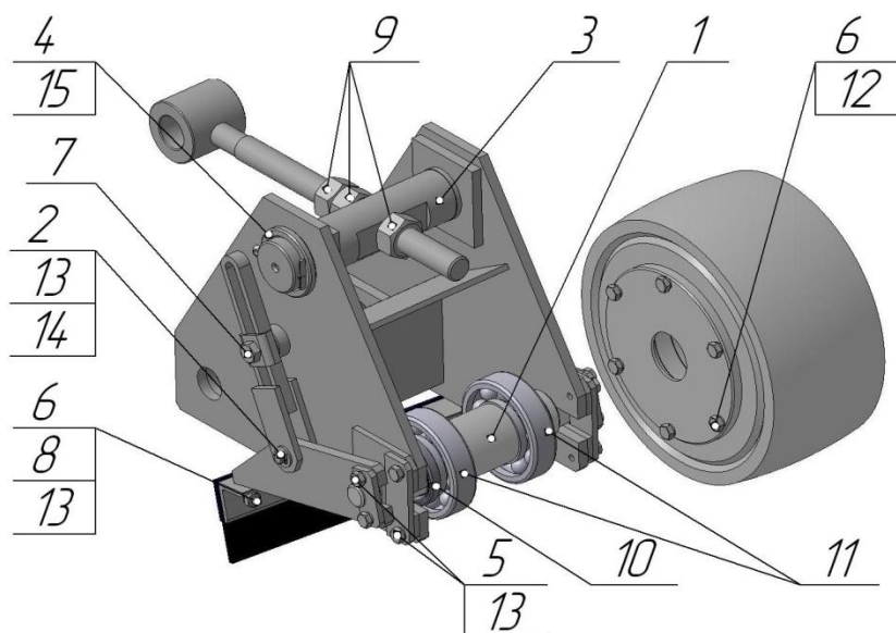
Рисунок 9. Колесо ФД-567.08
