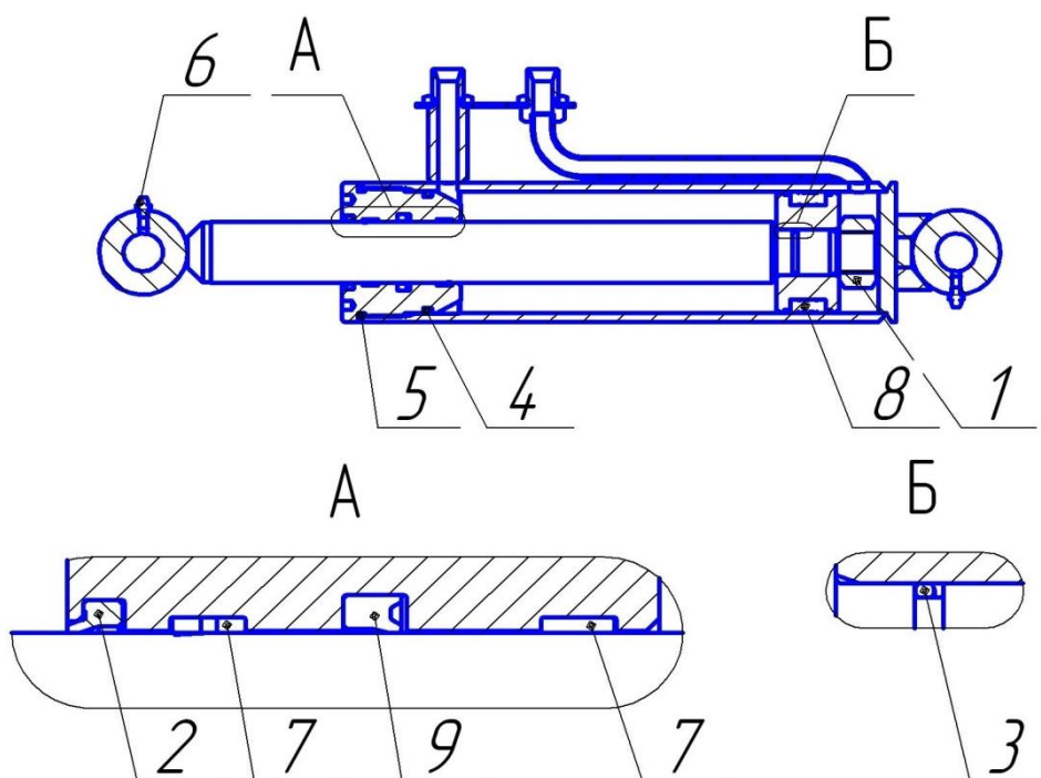
Рисунок 16. Гидроцилиндр ЦГ-ПМК-80.40.200.515-Е9-Р15-01
