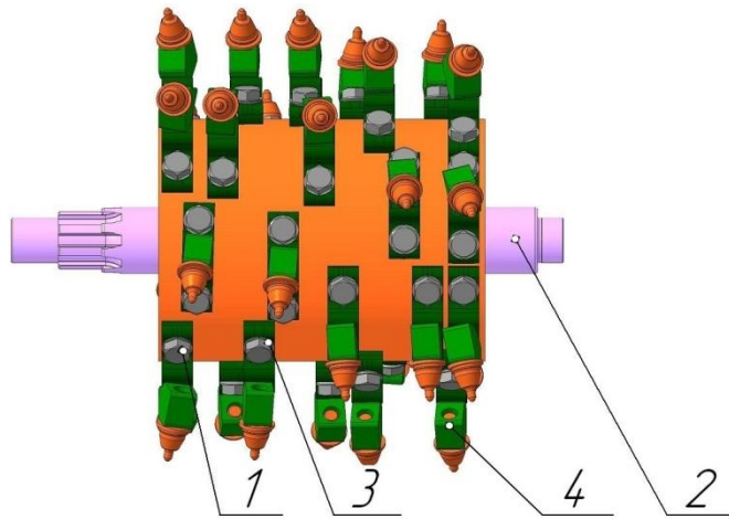
Рисунок 8. Фреза ФД-567.07
