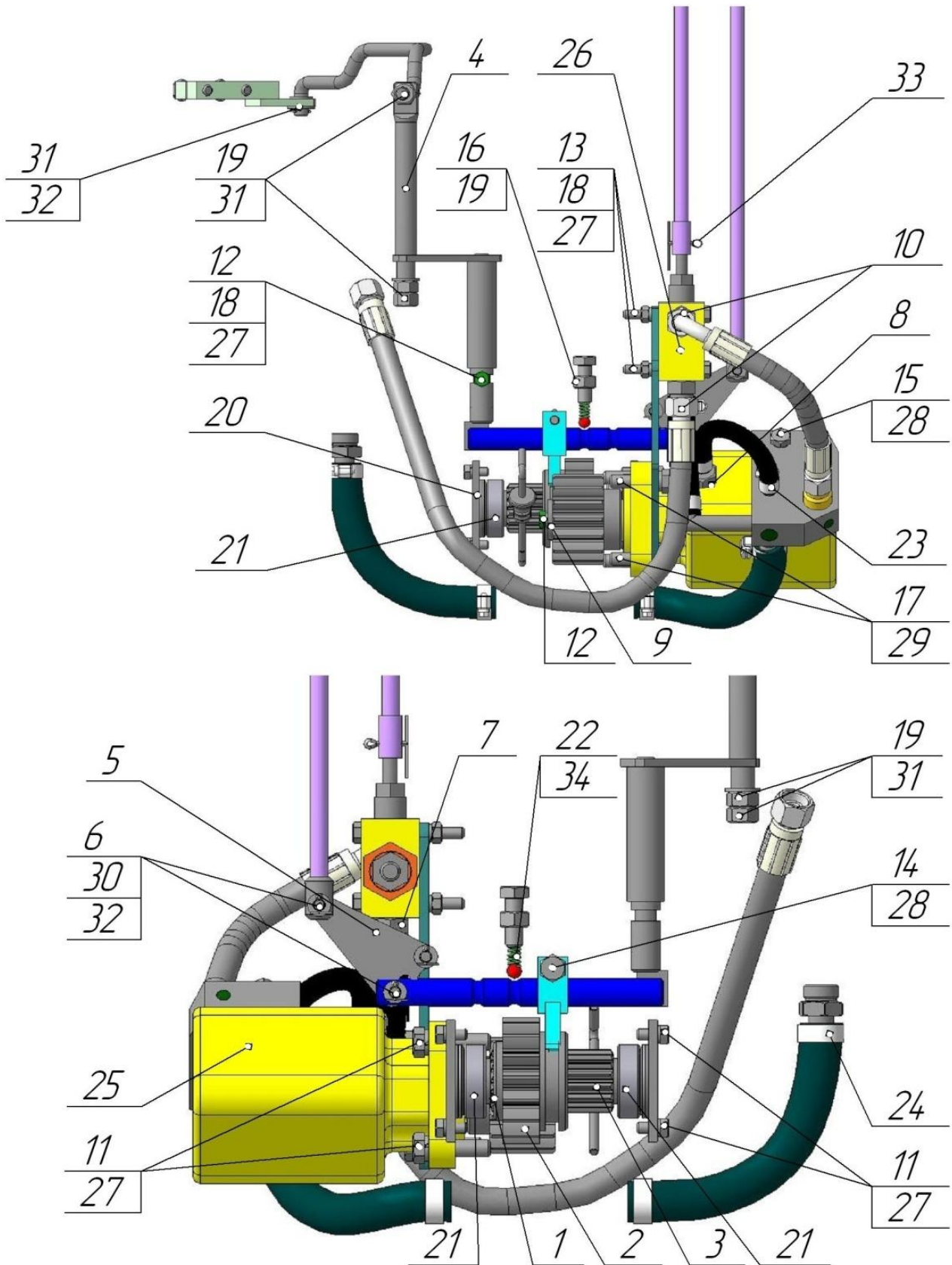
Рисунок 15. Гидроходоуменьшитель ФД-567.11
