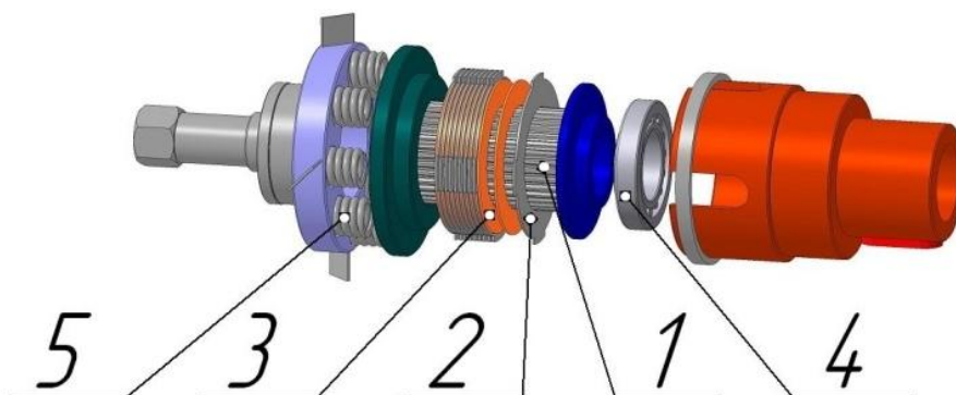
Рисунок 3. Муфта фрикционная ФД-567.01.02
