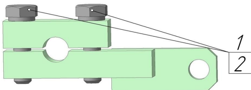
Рисунок 14. Хомут-567.11.10
