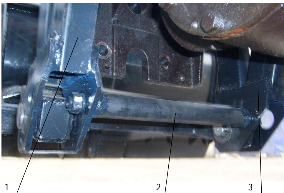
Рисунок 5. Сборка Подрамников.
