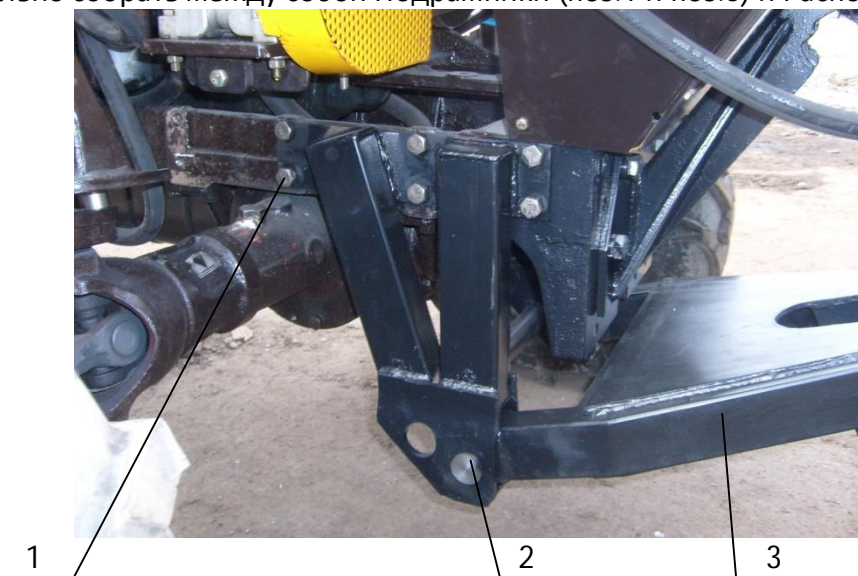
Рисунок 6. Установка Подрамников и Рамы.
