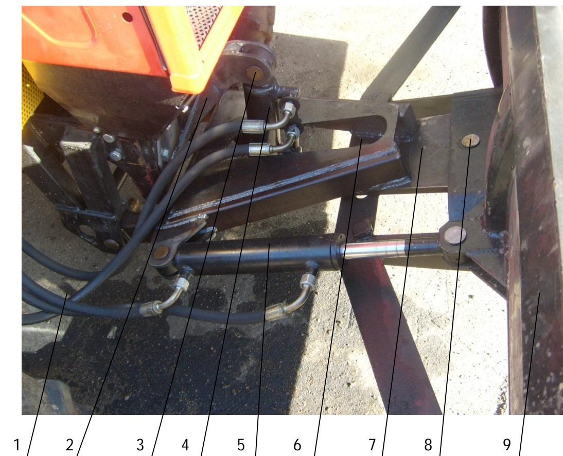
Рисунок 7. Установка Лопаты, Кронштейна и Гидроцилиндров подъема - опускания и поворота Лопаты.
